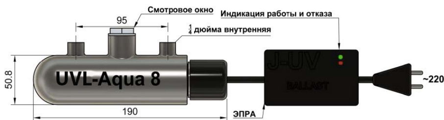
Рисунок 1. Габариты установки UVL -Aqua 8
