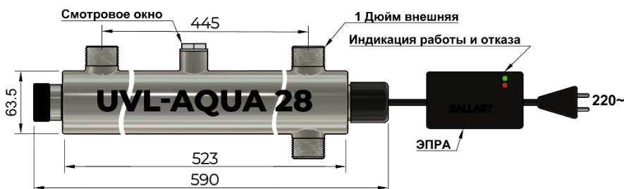
Рисунок 1. Габариты установки UVL-Aqua 28
