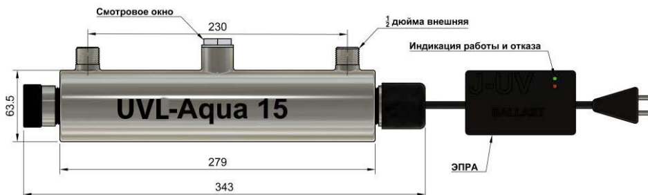
Рисунок 1. Габариты установки UVL-Aqua 15
